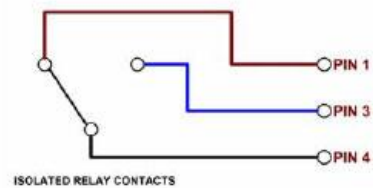
Funcionamiento del relé de monitorización remota.
